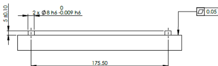
1.2: Montážní deska pro základnu robota
